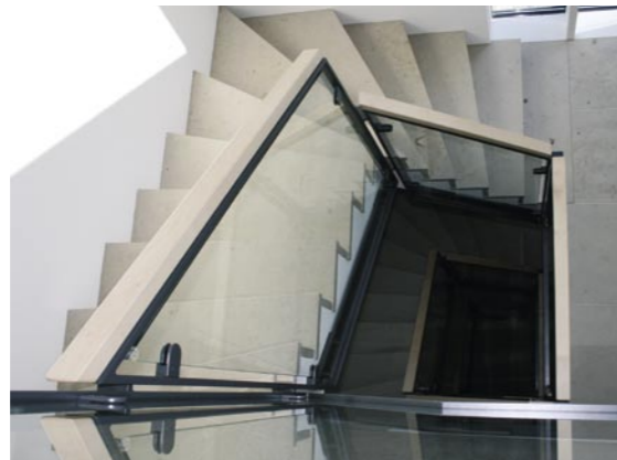
Treppengeländer aus Stahl, pulverbeschichtet mit Glasfüllung und Holzhandlauf
